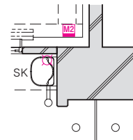
■ 15・16 階部分図
