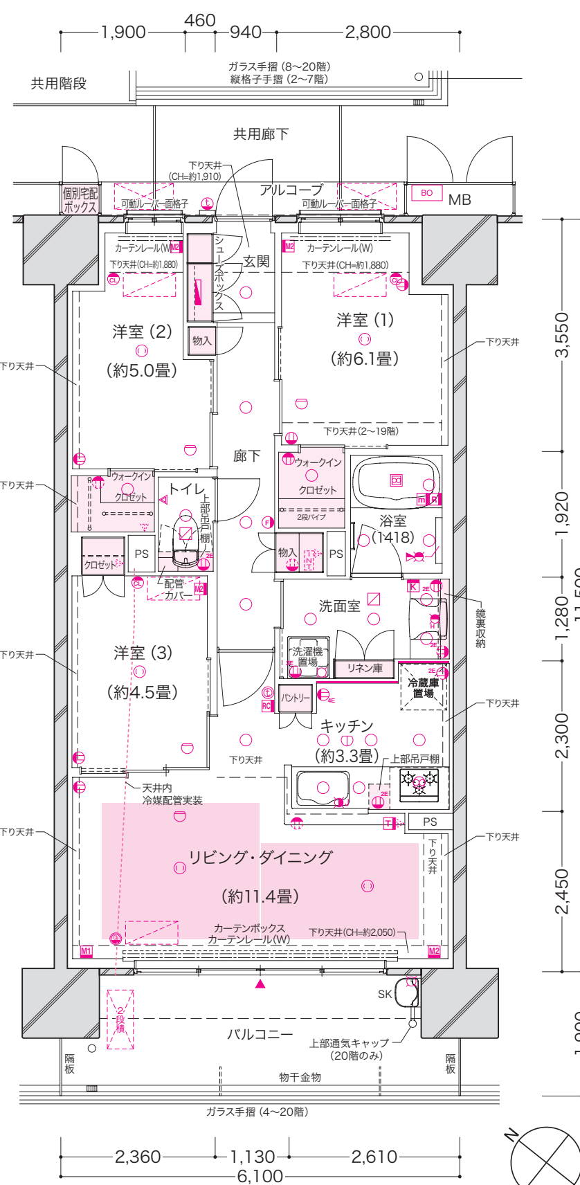
■ 2・3 階部分図
