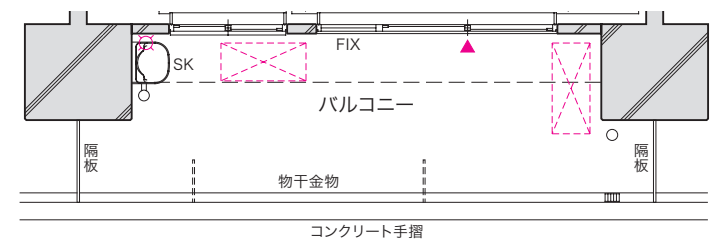
■ 2・3 階部分図
