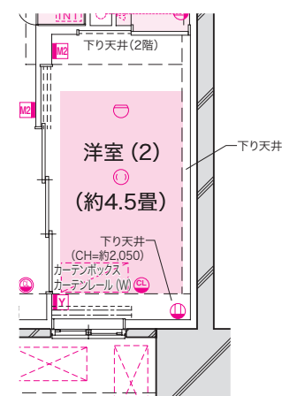
■ 2・20 階部分図
