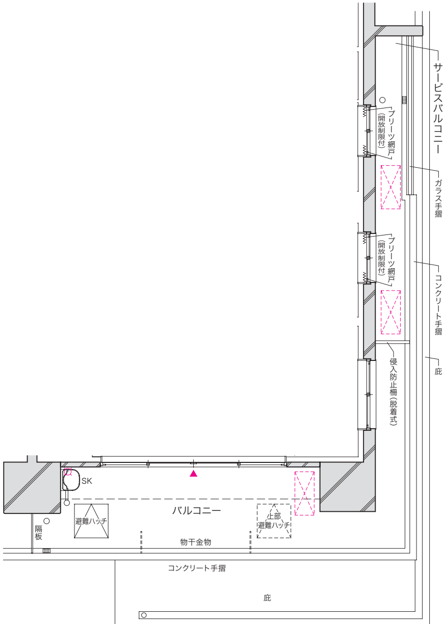
■ 3 階部分区
