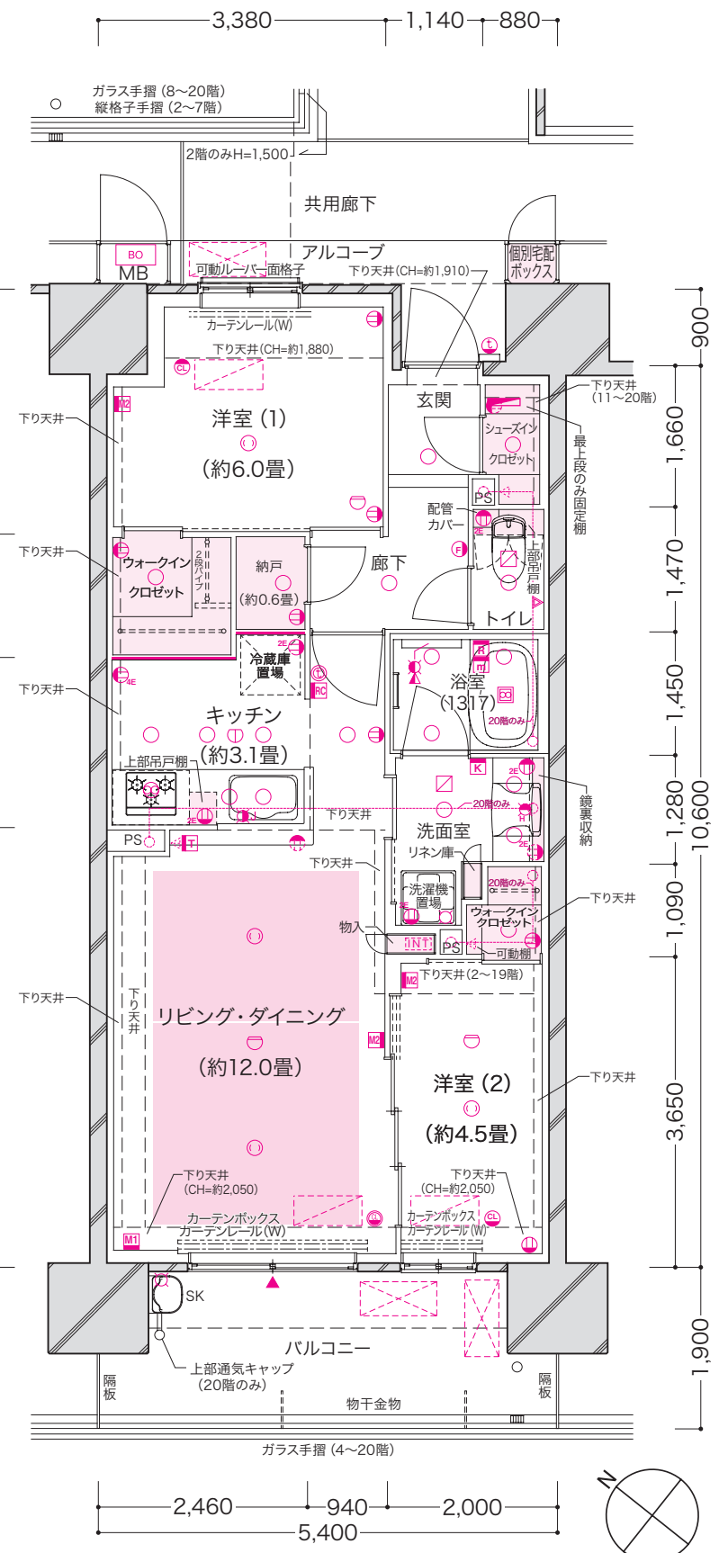
■ 2・3 階部分図
