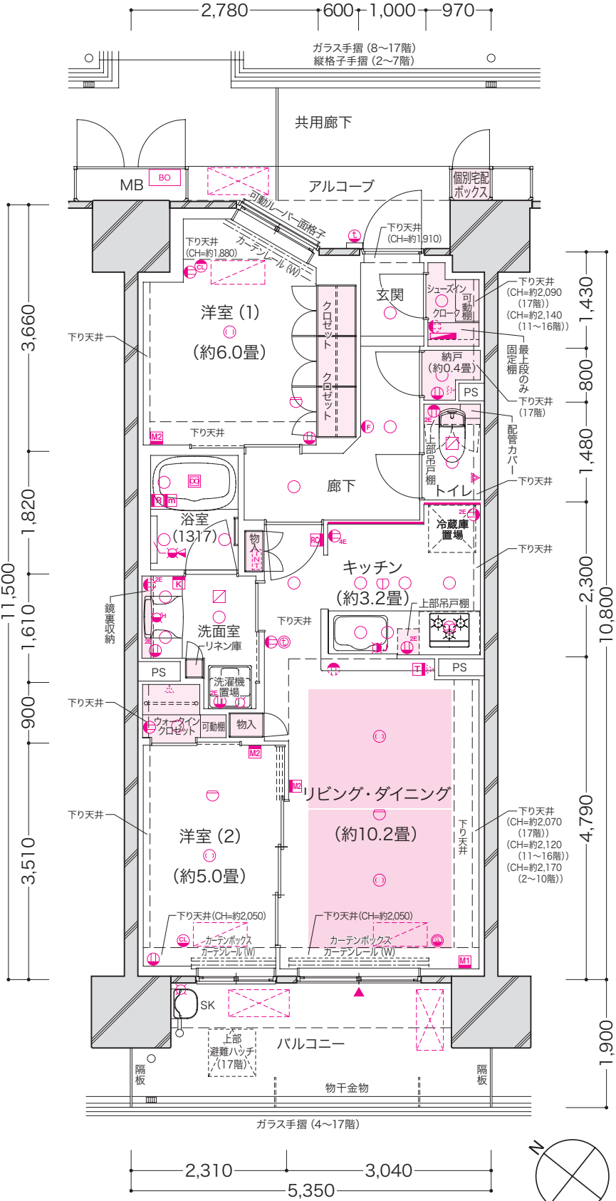
■ 15・16 階部分図
