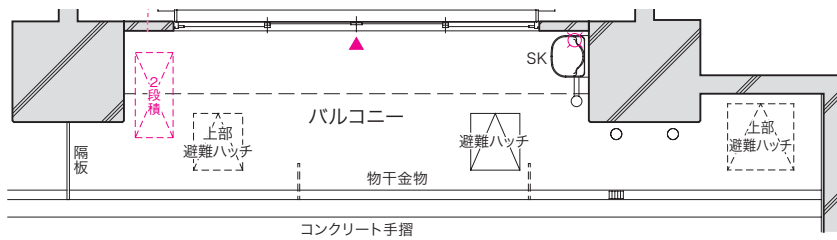
■ 2 階部分図
