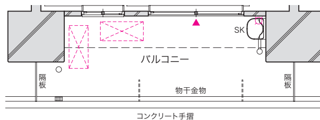
■ 2・3 階部分図
