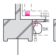
■ 15・16 階部分図
