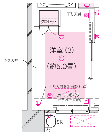
■ 2 階部分図
