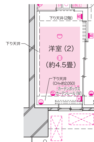
■ 2・20 階部分図
