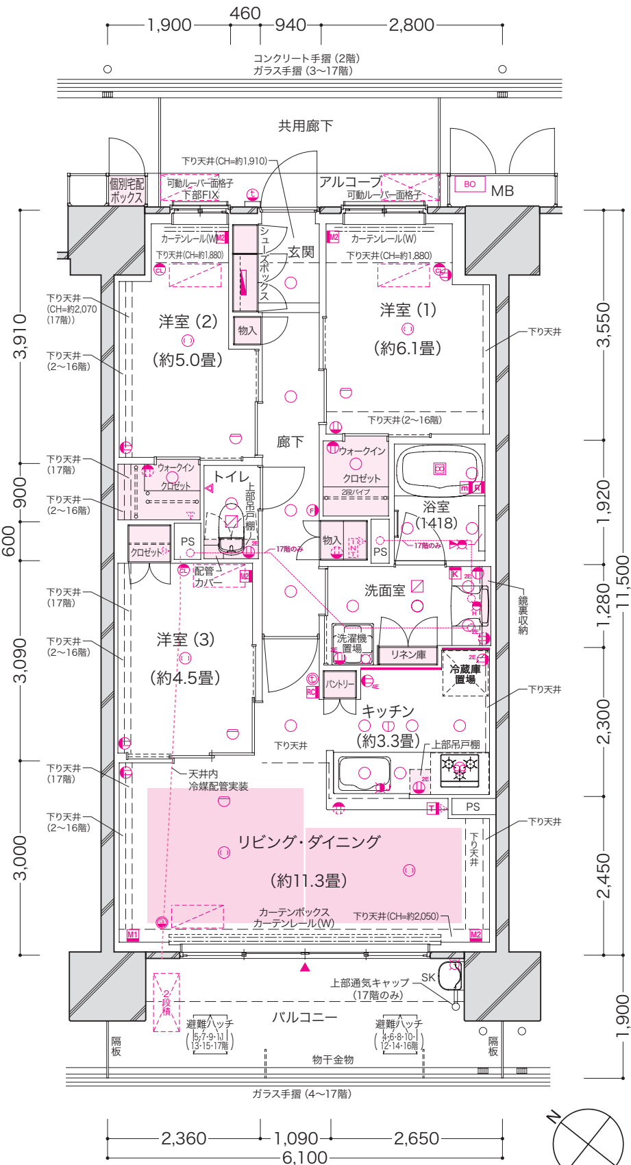
■ 15・16 階部分図
