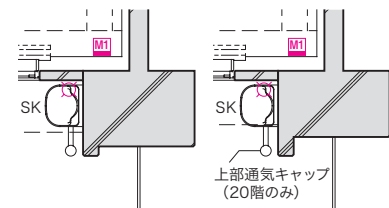
■ 15・16 階部分図
