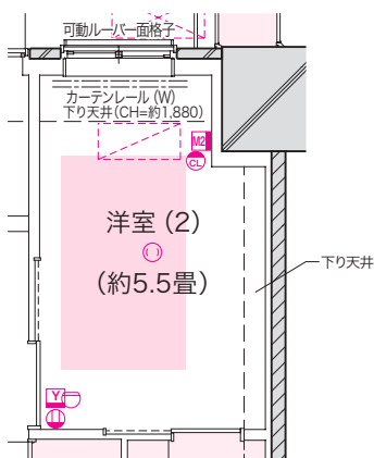
■ 2 階部分図
