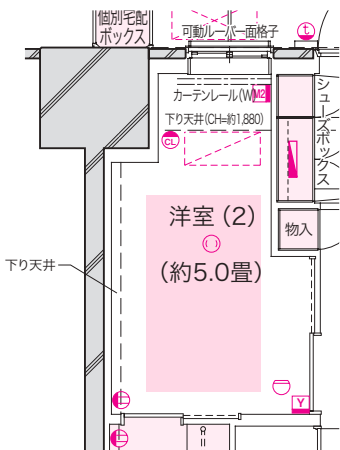
■ 2・20 階部分図
