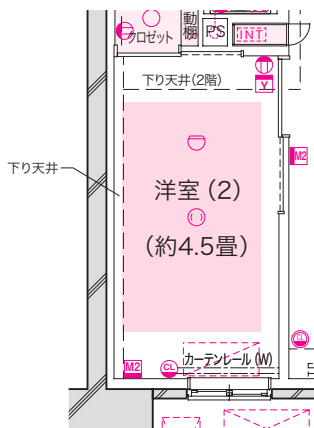
■ 2・20 階部分図
