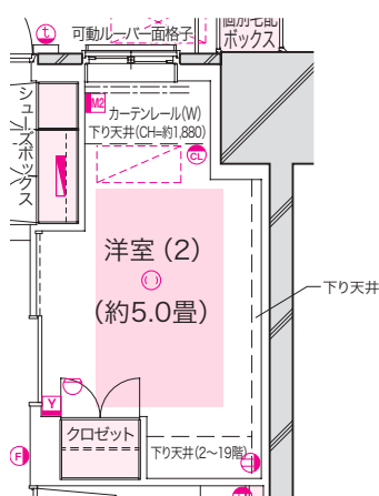
■ 20 階部分図
