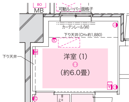
■ 2・20 階部分図
