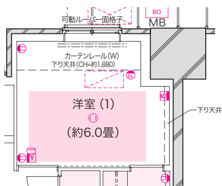
■ 2・20 階部分図
