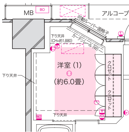
■ 2・20 階部分図
